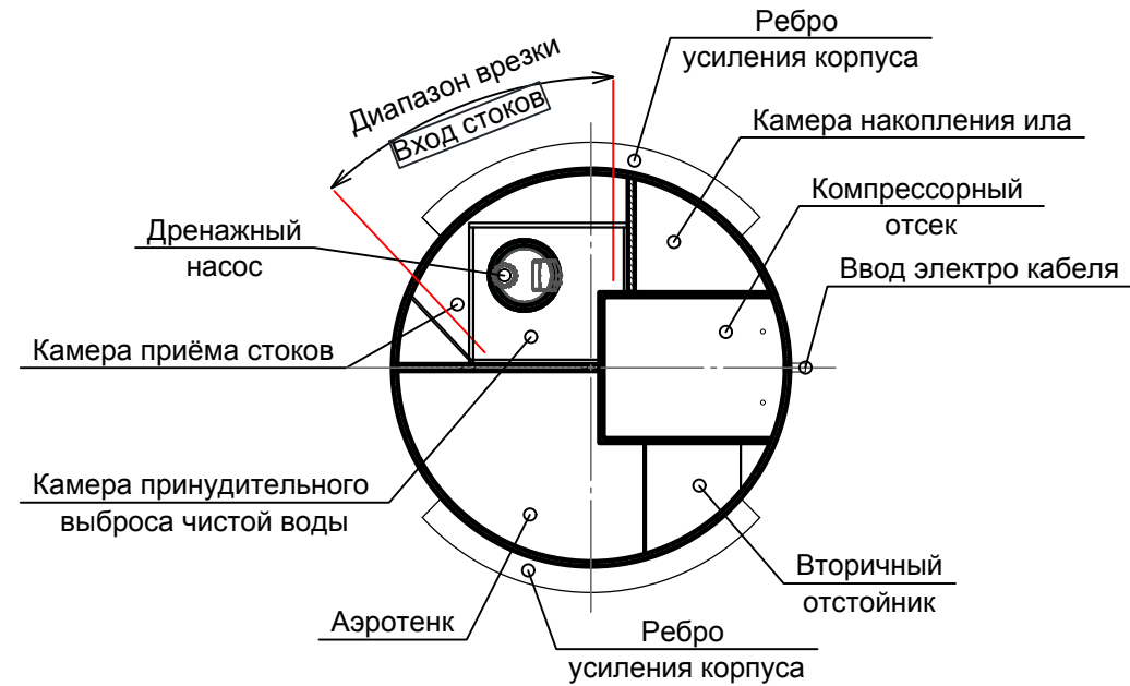
Схема расположений камер
