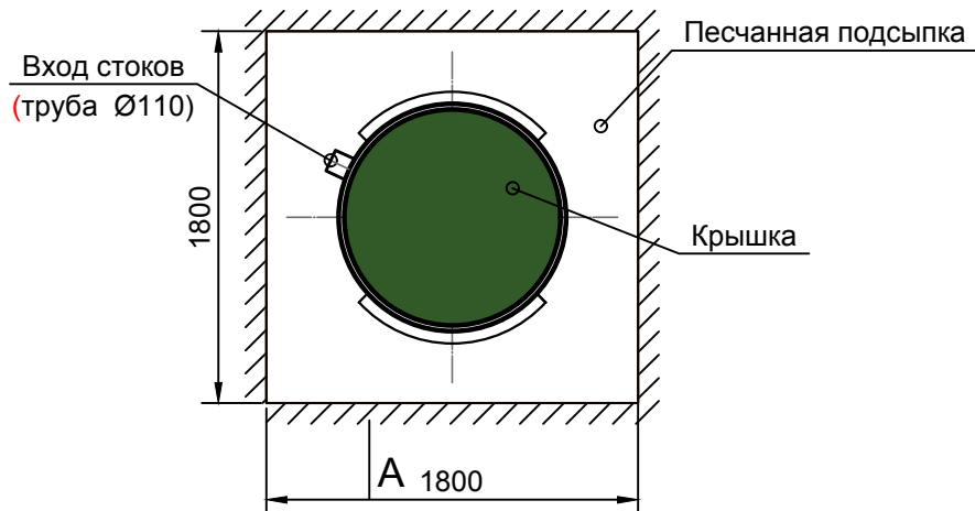
Вид сверху
